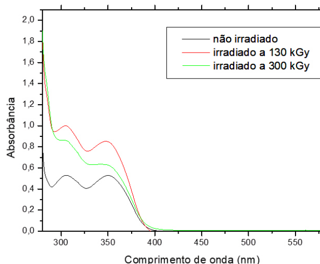
Fig. 5: Curvas de absorbância obtidas por espectrofotometria UV/VIS para as amostras não irradiada e irradiadas com doses de 130 kGy e 300 kGy
