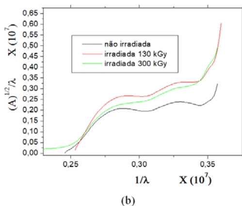
Fig. 6: Curvas \frac{\sqrt{A}}{\lambda} vs \frac{1}{\lambda} para as amostras não irradiada e irradiadas por radiação ultravioleta (a) e gama (b)
