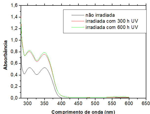
Fig. 4: Curvas de absorbância obtidas por espectrofotometria UV/VIS para as amostras não irradiadas e expostas a 300 h e 600 h de radiação ultravioleta
