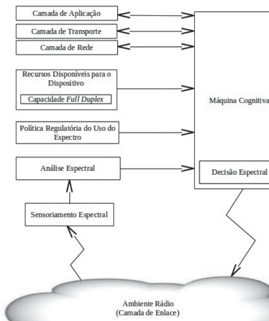
Fig. 10 – Arquitetura para Nós Cognitivos em Redes Táticas Sem Fios.
