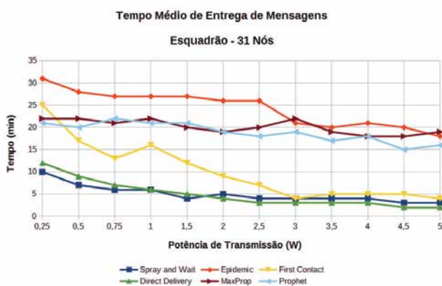
Fig. 8 – Tempo Médio de Entrega de Mensagens
