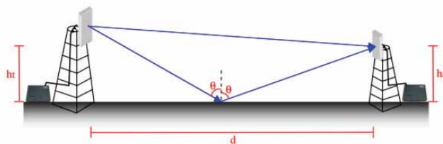
Fig. 5 – Modelo de Propagação de 2 raios [27]
