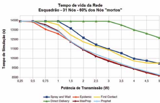
Fig. 6 – Tempo de Vida da Rede
