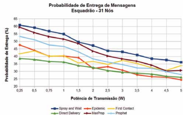
Fig. 7 – Probabilidade de Entrega de Mensagens
